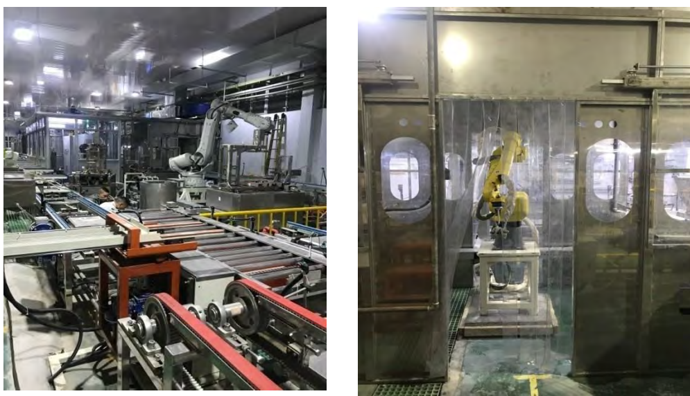
圖、機器人噴釉系統
